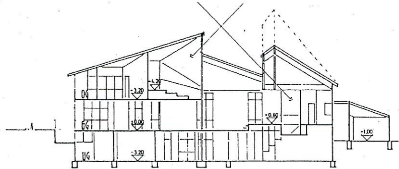
SCHNITT C-D
