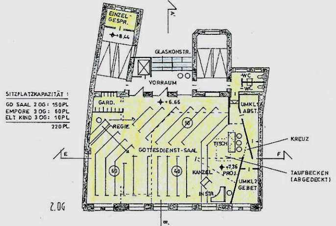
3.OG
