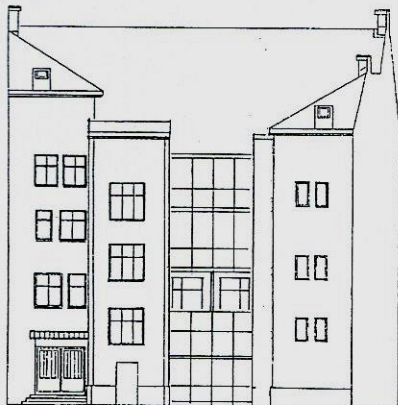
HOFANSICHT
