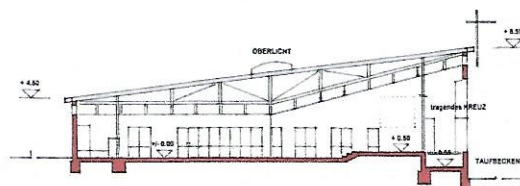
SCHNITT B - B
